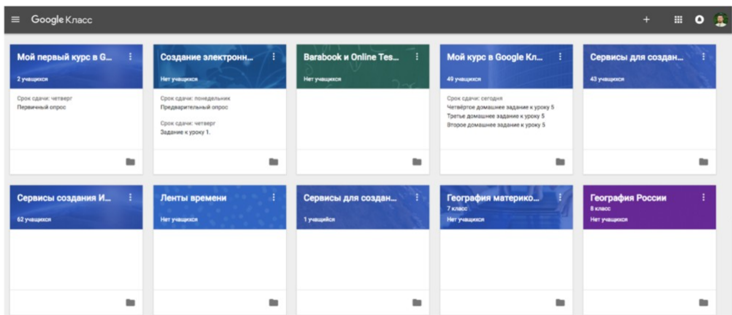
Рисунок 2. Google Класс
